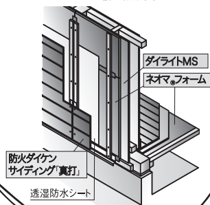
「外張りDNシステム」構造説明図
